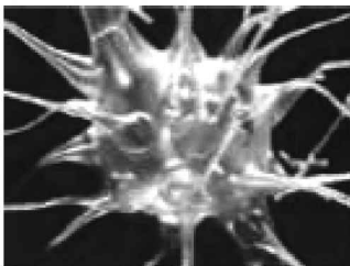
Sel Otak
